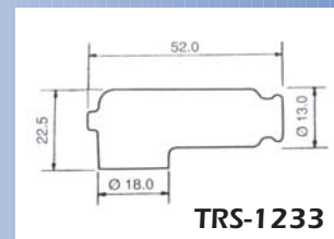
Universal Kerzenstecker (Speziell alte Kawasaki) Metall 5K-OHM Bestell-Nr. 50347820
