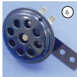
1) 6V schwarz, ø90mm Bestell-Nr. 7618016 12V schwarz, ø90mm Bestell-Nr. 7618022
